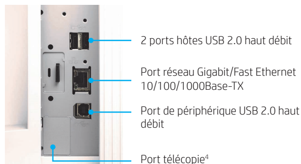
Gros plan du panneau d'E/S arrière
